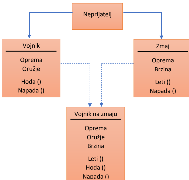
Slika 2. Struktura entiteta nakon dodavanja entiteta vojnik na zmaj
