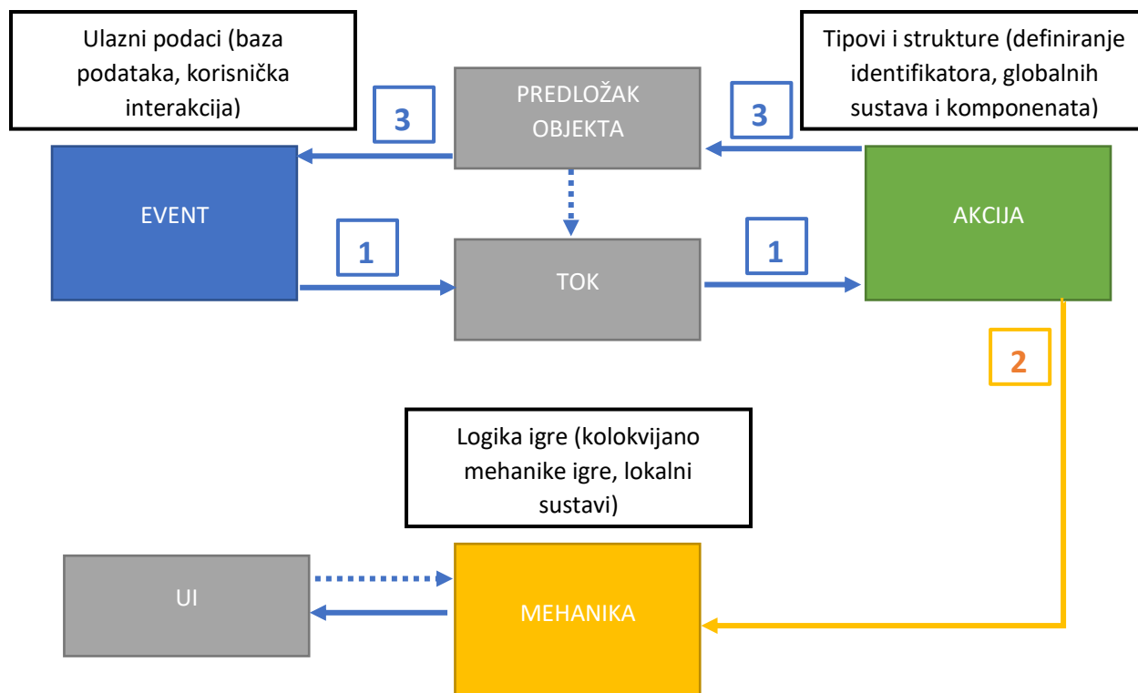
Slika 9. Apstraktni prikaz izvođenja igre pri interakciji korisnika
