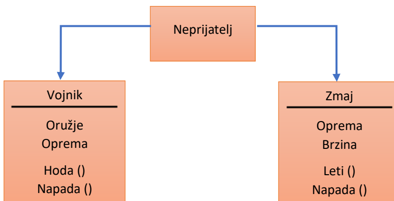
Slika 1. Struktura nekih entiteta u objektno orijentiranom dizajnu
