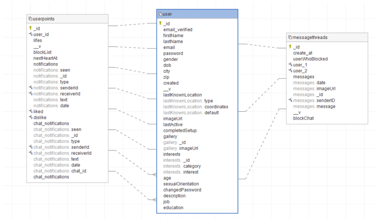
Slika 2. ER dijagram baze podataka
