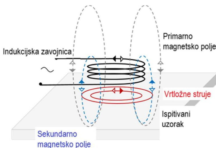
Slika 38. Način rada ispitivanja zavarenog spoja pomoću vrtložnih struja
