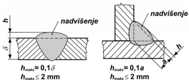
Slika 15. Primjeri prevelikog nadvišenja zavara
