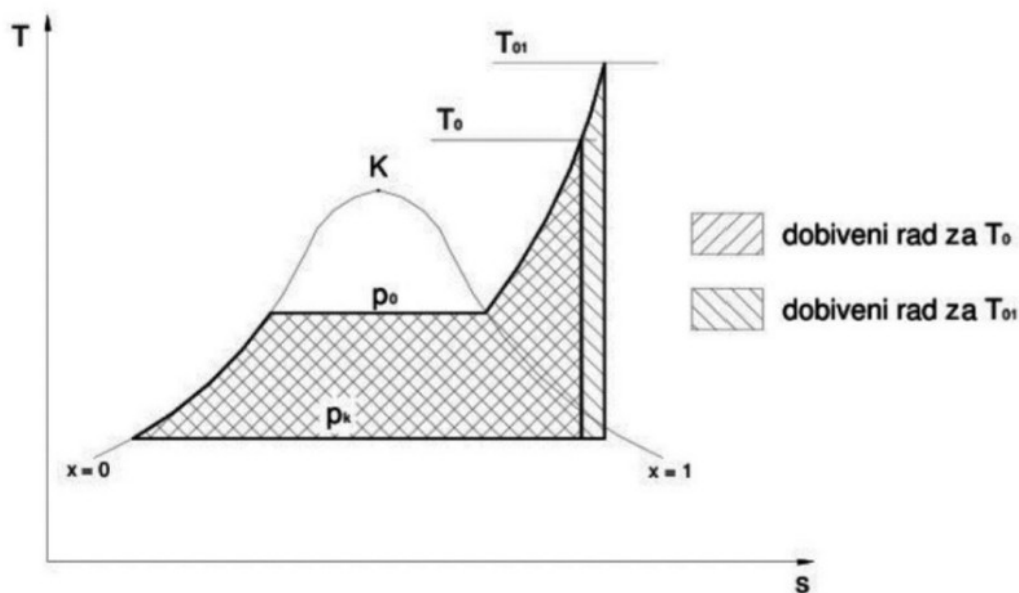
Slika 15. T-s dijagram podizanja temperature svježeg pare [8]
