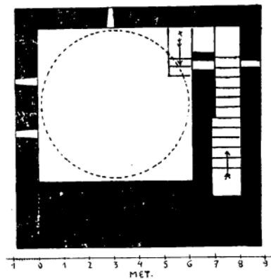
SI 37. Horizontalni presjek prvog kata barutane Mazalić, 1952. str. 77
