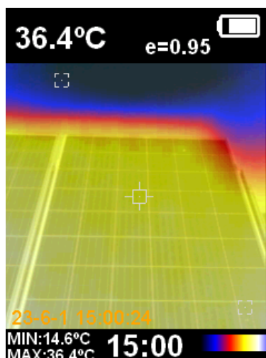
Slika 45. Temperatura na panelu broj 4
