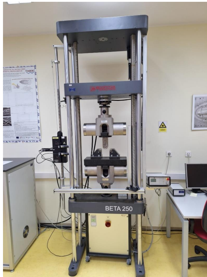
Slika 14: Univerzalnoj statička kidalica BETA250, tvrtke Messphysik
