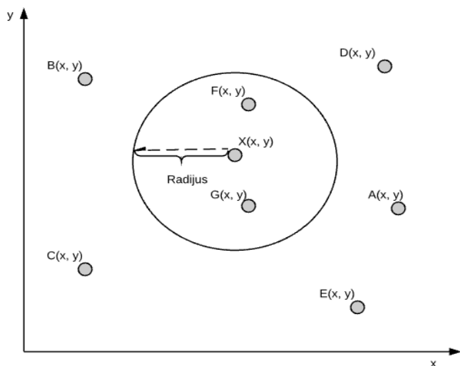
Slika 6. Geometrijska interpretacija pojasa sličnosti 33
