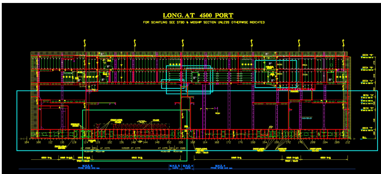
Slika 4: Prikaz plana željeza za longitidine
