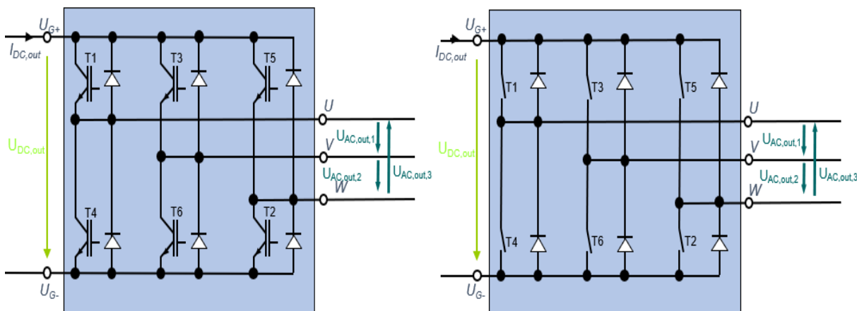
Slika 19. Izmjenjivač [14]
