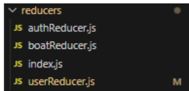
Slika 31 Reducers direktorij
