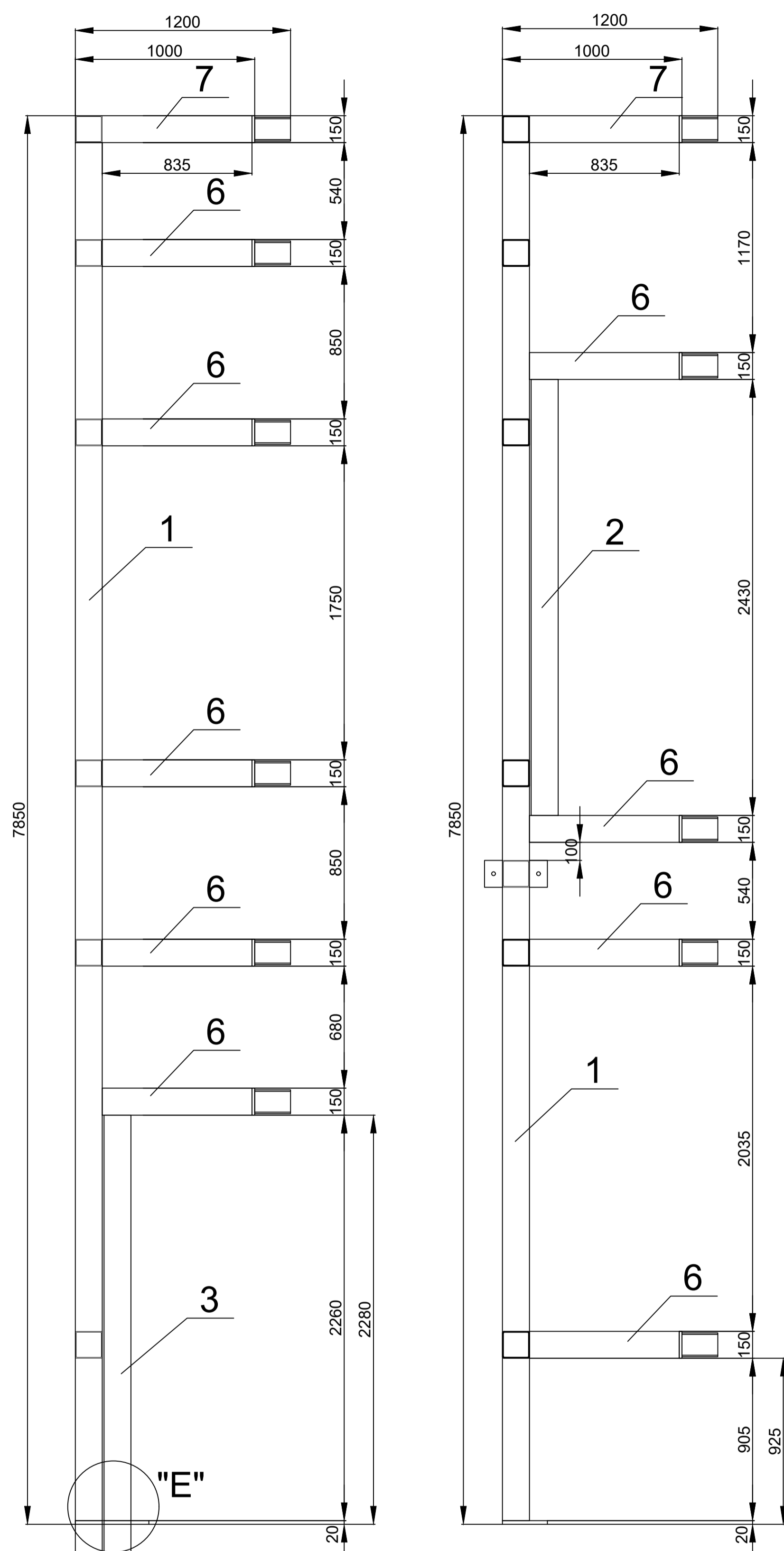
POGLED "A"
