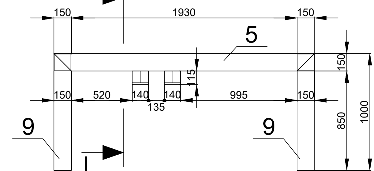
POGLED "C"
