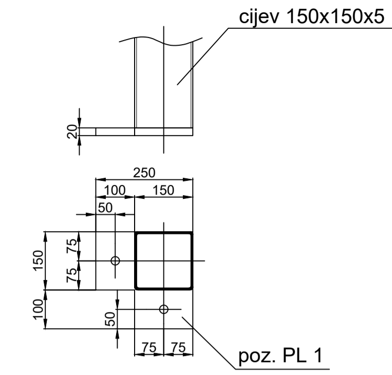
DETALJ "F"
