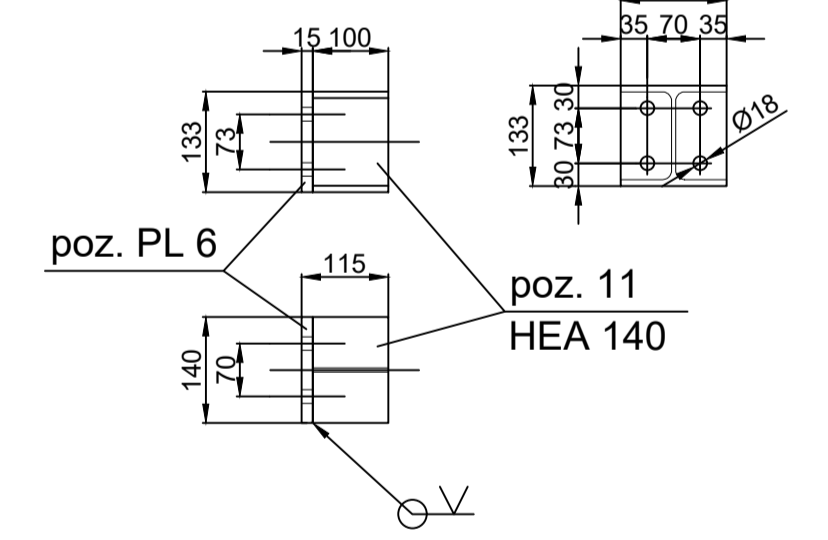
POZICIJA 11 HEA160 - sklop M1:10
