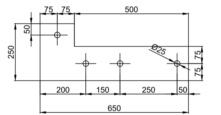
PL3 250 X 650 X 20 kom 1
