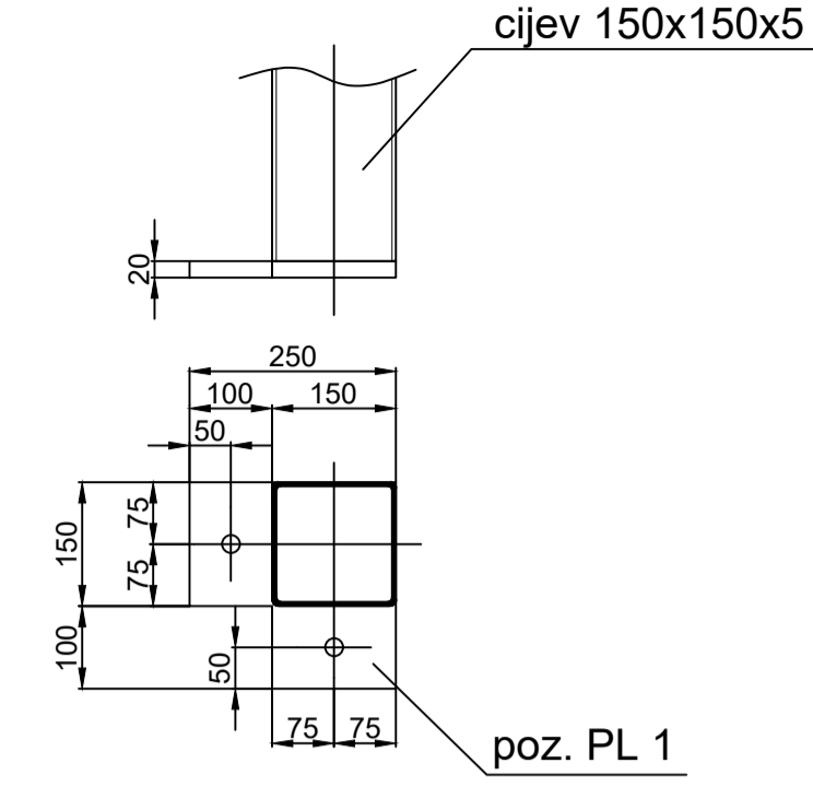
DETALJ "F" M1:10
