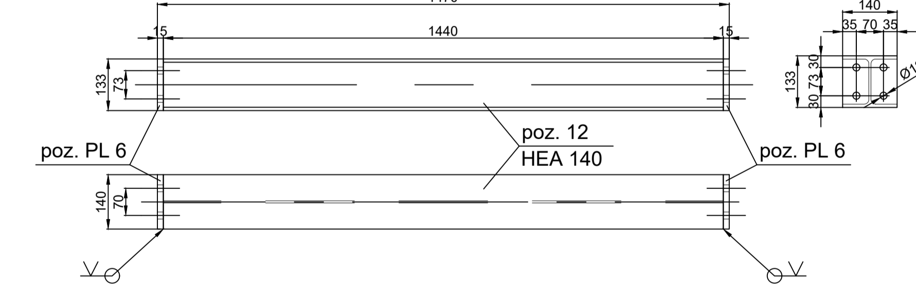
DETALJ SPOJA SEKCIJA 1 i 2
