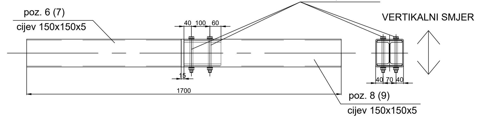
DETALJ SPOJA SEKCIJA 1 i 2 M1:10
