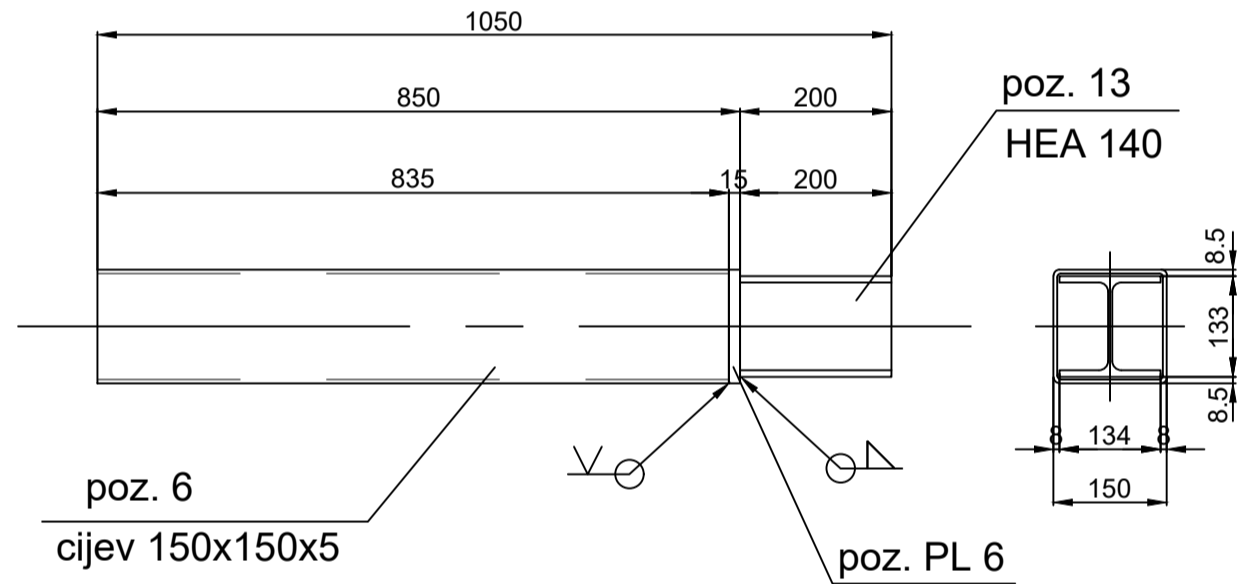
POZICIJA 6 cijev 150 x 150 x 5 - sklop M1:10
