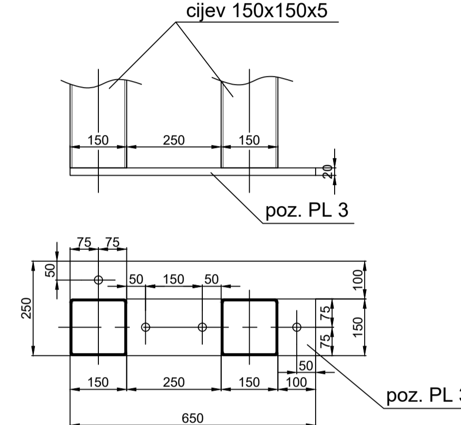
POZICIJA 6 cijev 150 x 150 x 5 - sklop
