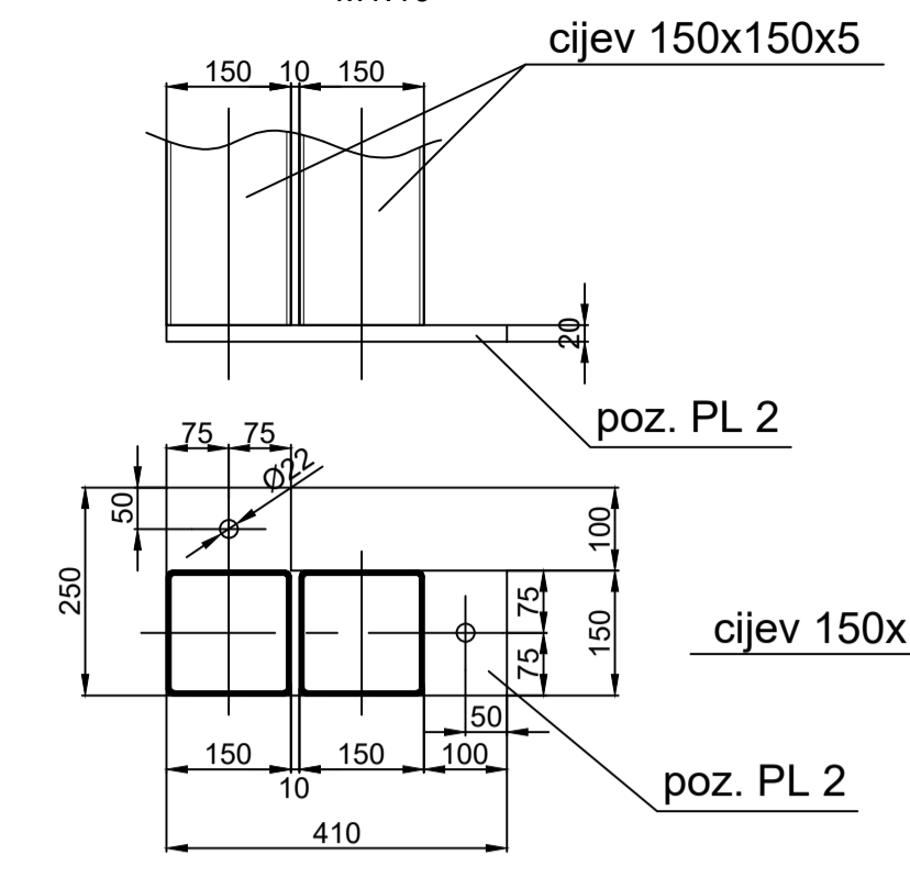
DETALJ "E" M1:10
