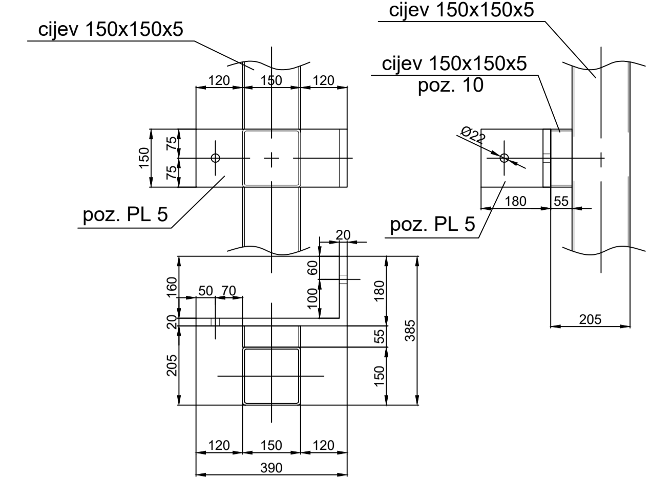
PRESJEK I - I
