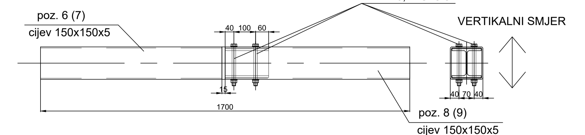
DETALJ SPOJA SEKCIJA 1 i 2
