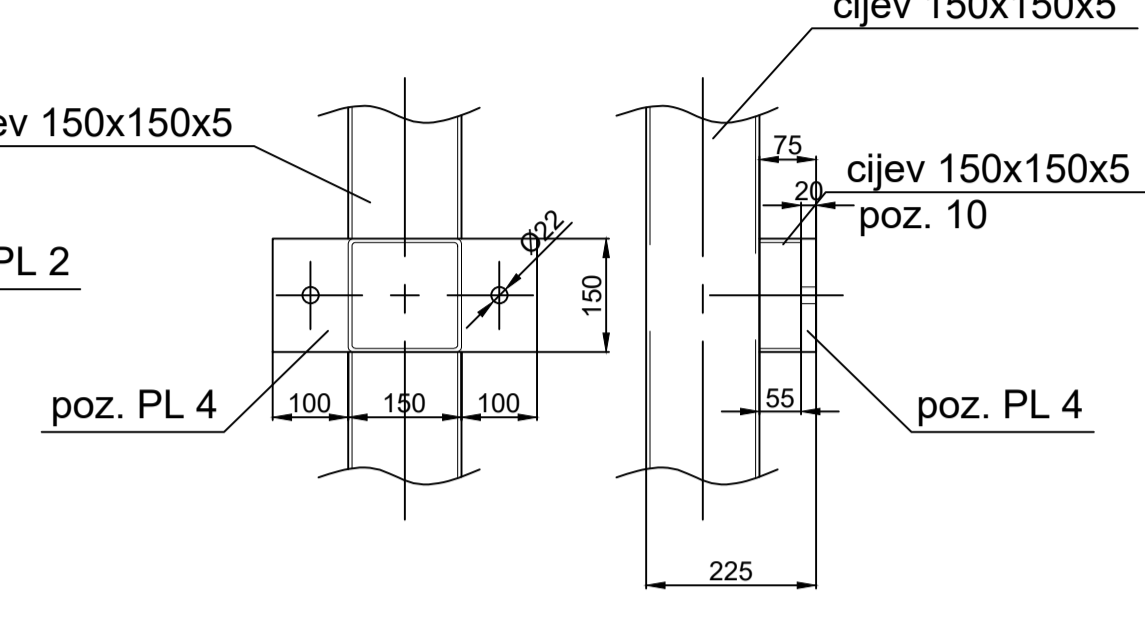
DETALJ "G" M1:10
