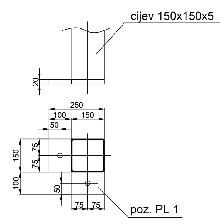
DETALJ "D" M1:10
