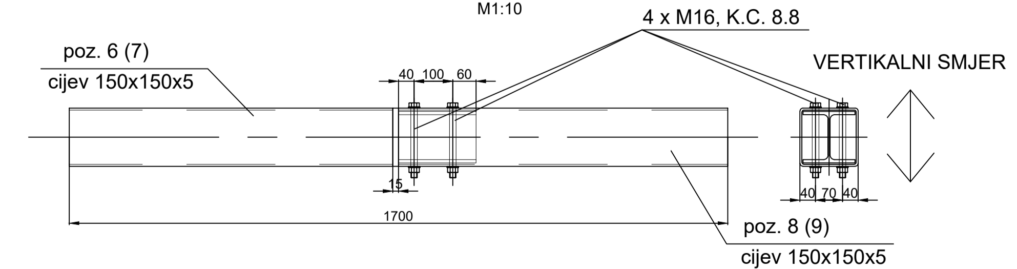
DETALJ SPOJA SEKCIJA 1 i 2 M1:10
