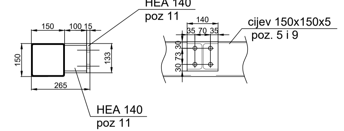
PRESJEK I - I M1:10
