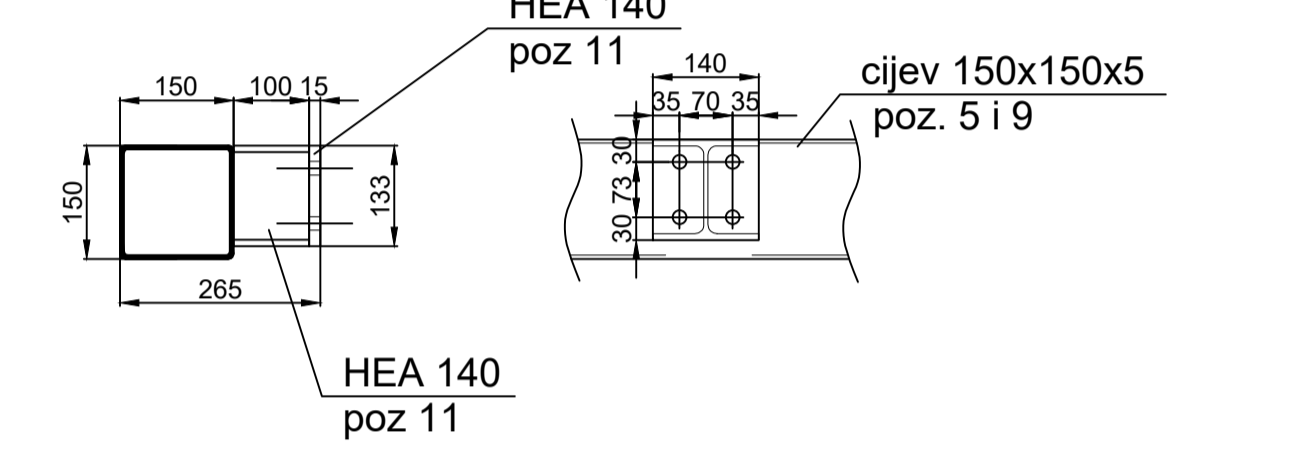
PRESJEK I - I M1:10
