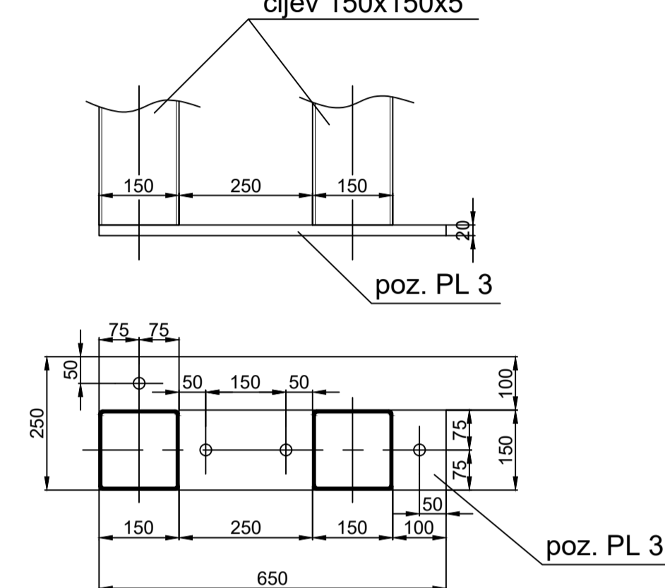
POZICIJA 6 cijev 150 x150 x 5 - sklop M1:10
