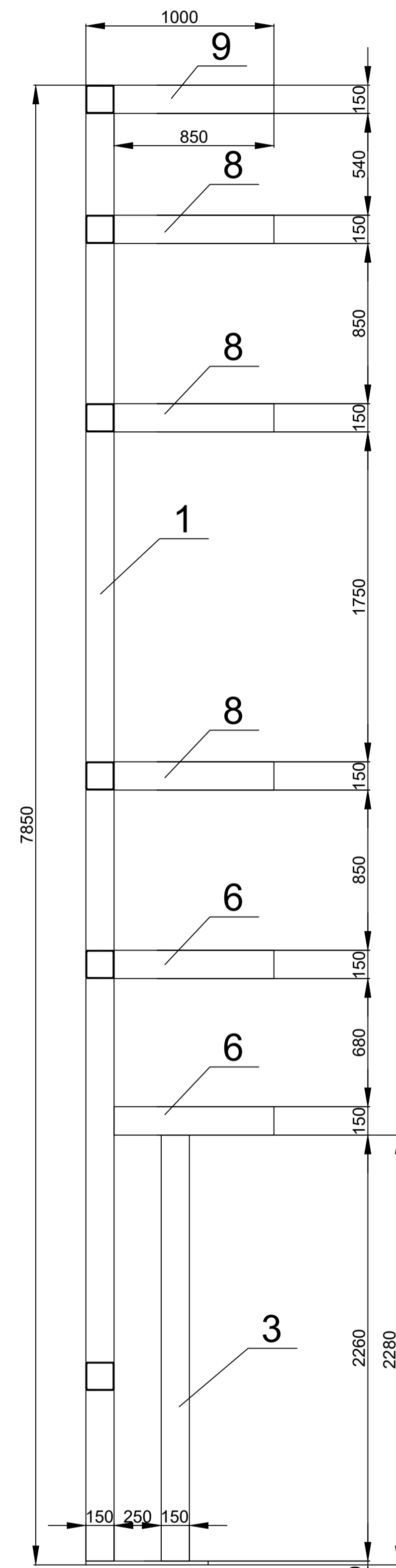
PRESJEK B - B
