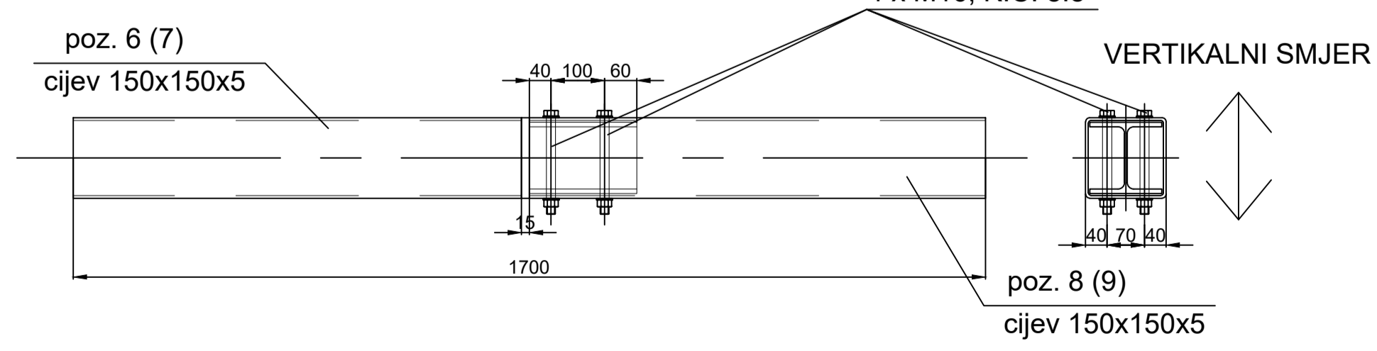
DETALJ SPOJA SEKCIJA 1 i 2 M1:10
