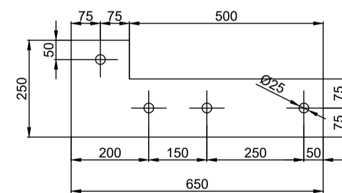
PL3 250 X 650 X 20 kom 1
