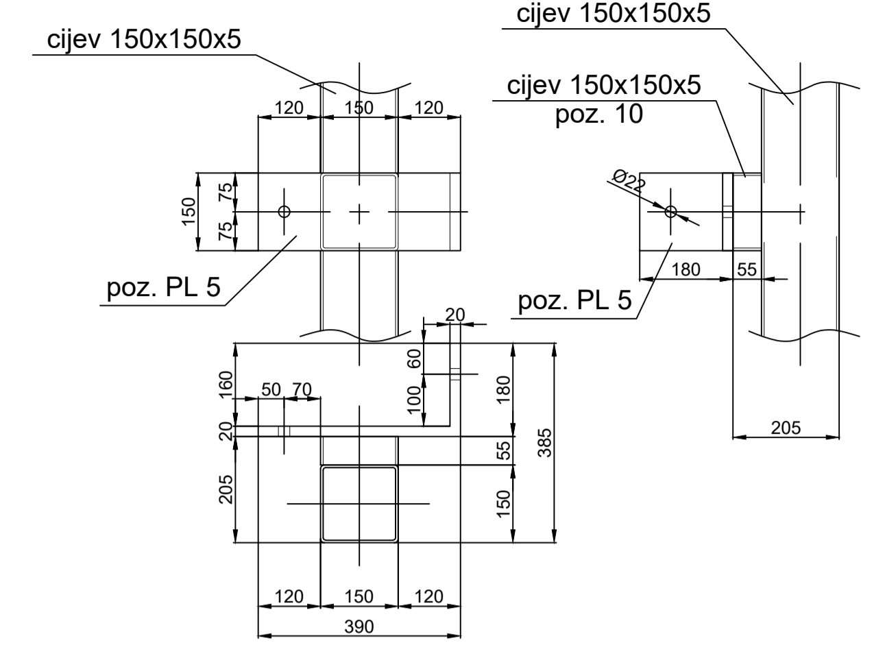
PRESJEK I - I M1:10
