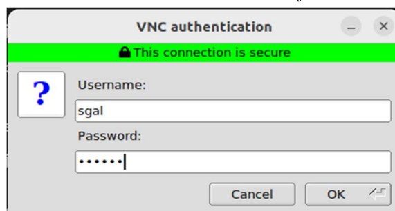
Slika 35: VNC autentifikacija
