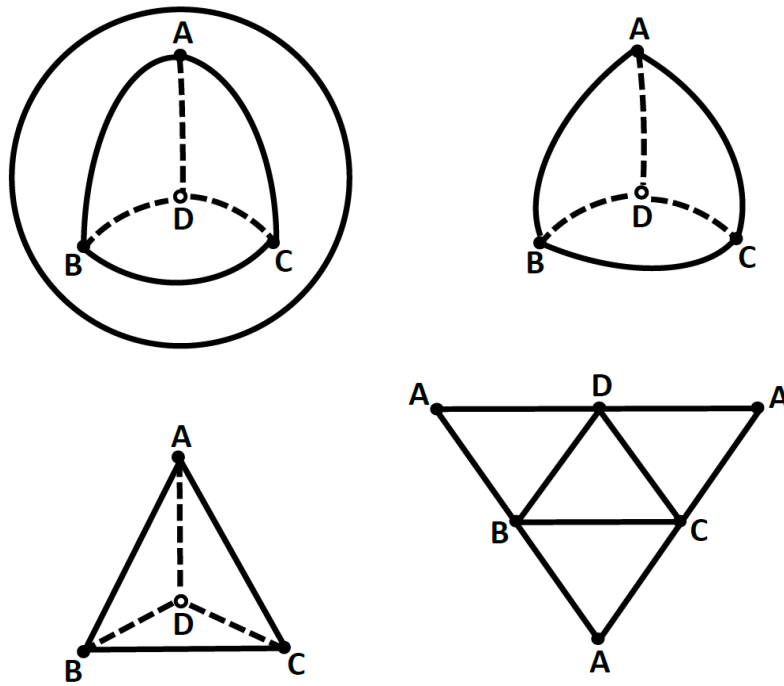
Slika 1 Trijagulacija 2-sfere
