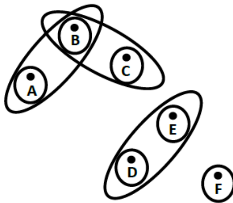
Slika 11 Simplicijalni kompleks
