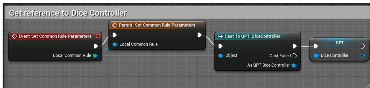
Slika 31. Funkcija SetCommonRuleParameters() u klasi DiceWithBoxTemplate.
