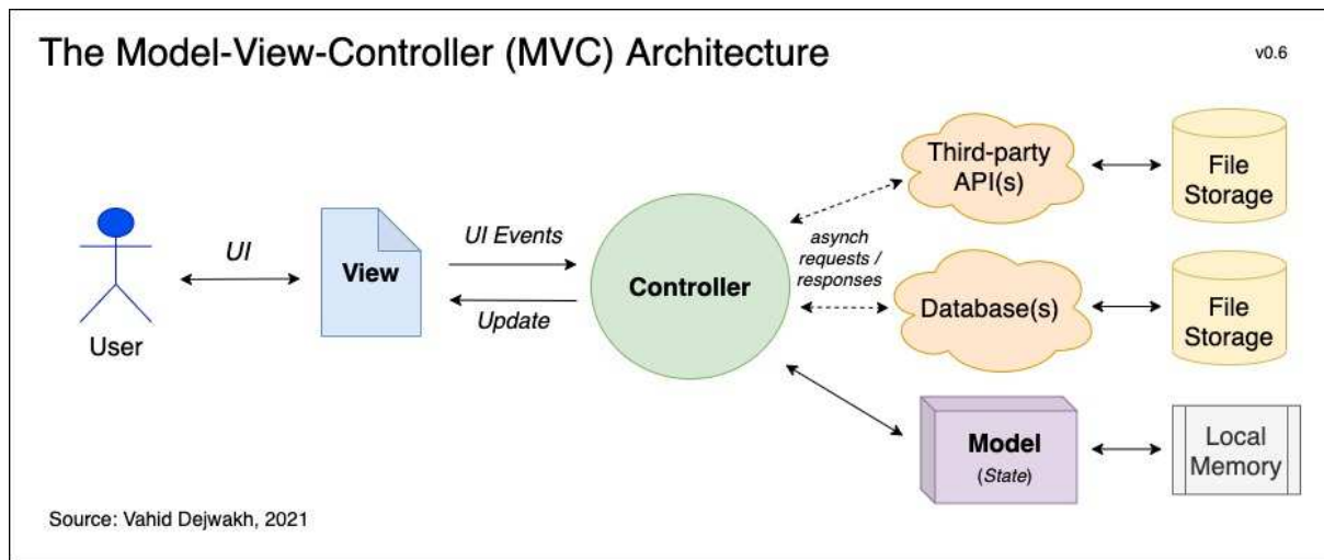
Slika 3. Prikaz MVC Arhitekture[8]
