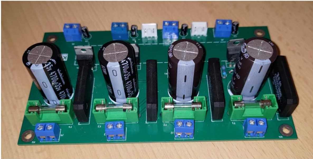
Slika 43: Gotova PCB pločica
