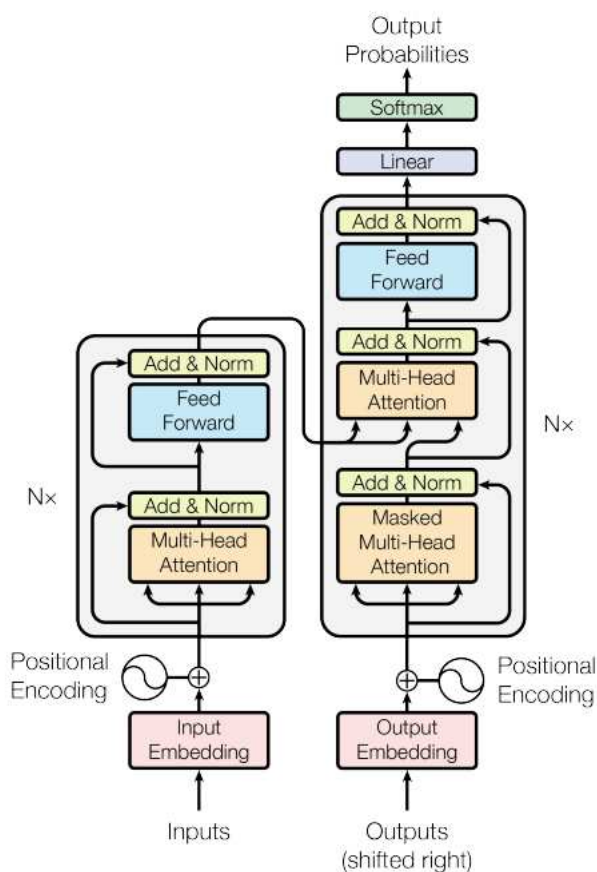
Slika 6: Arhitektura transformera [35]
