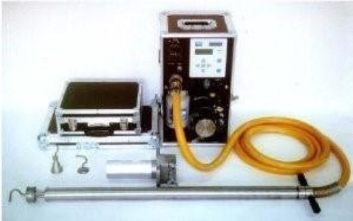
Slika 11. Mjerni uređaj SICK AG
