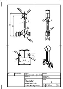
Slika 1.2: Primjer kotiranog nacrtu, klipnjača
