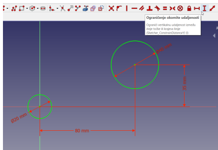
Slika 3.30: Prikaz izrade druge kružnice i definiranje njezina ograničenja
