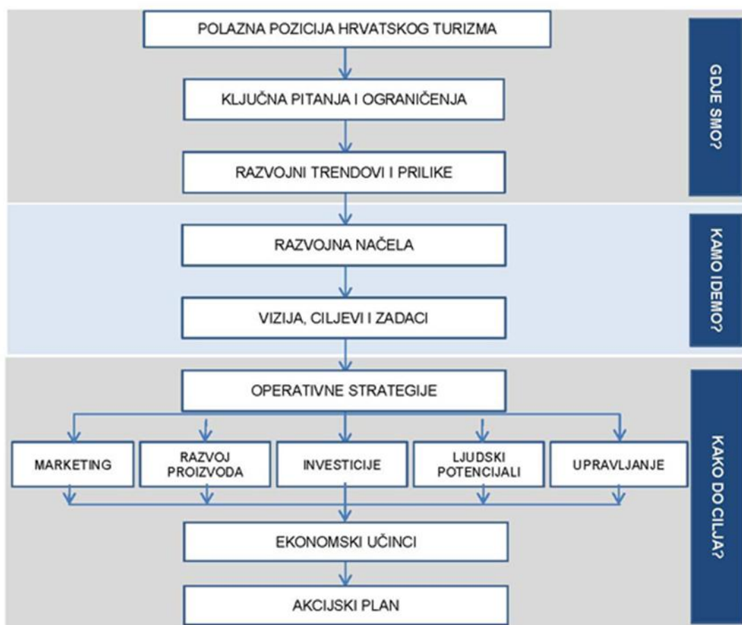
Slika 4. Struktura dokumenta
