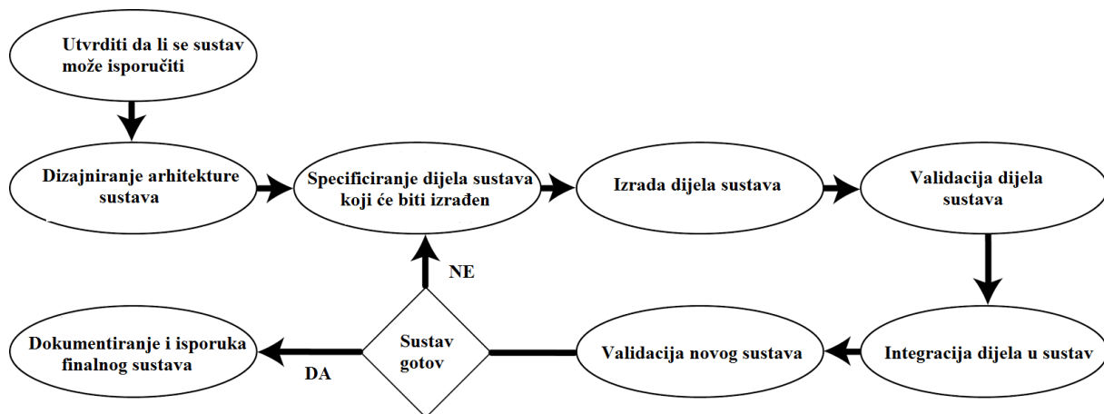
Slika 12. Inkrementalni razvoj
