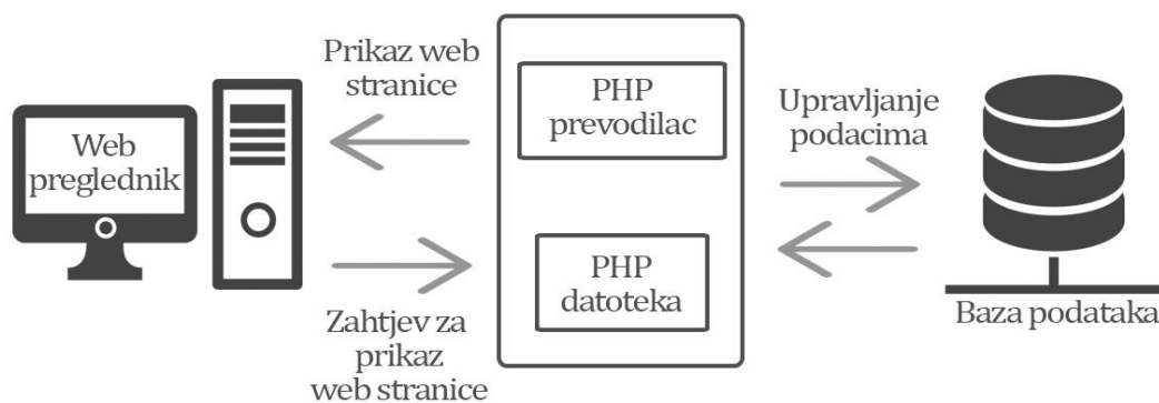
Slika 1. Povezivanje komponenti
