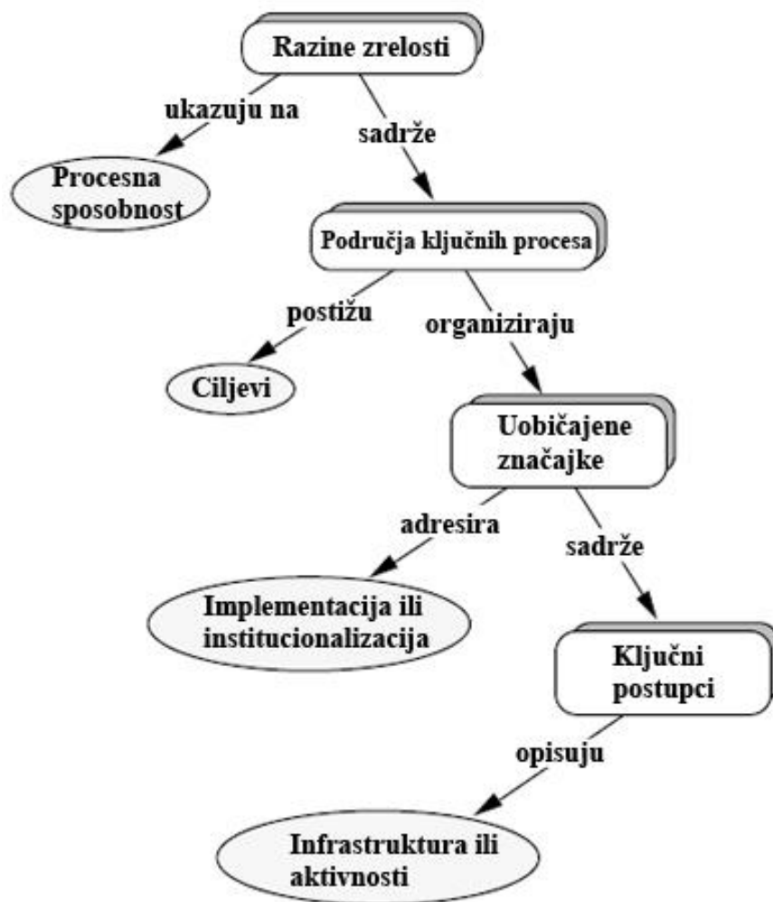
Slika 6. CMM struktura 22
