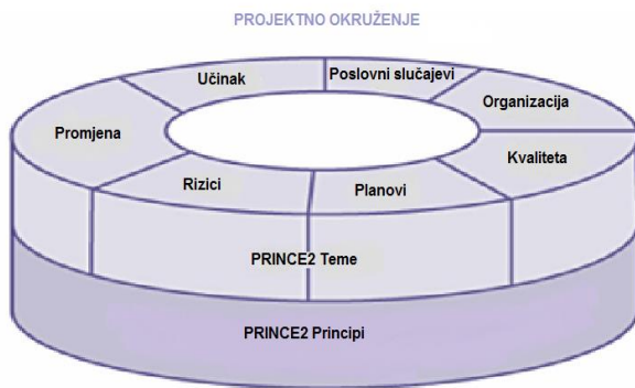
Slika 17: Struktura PRINCE 2
