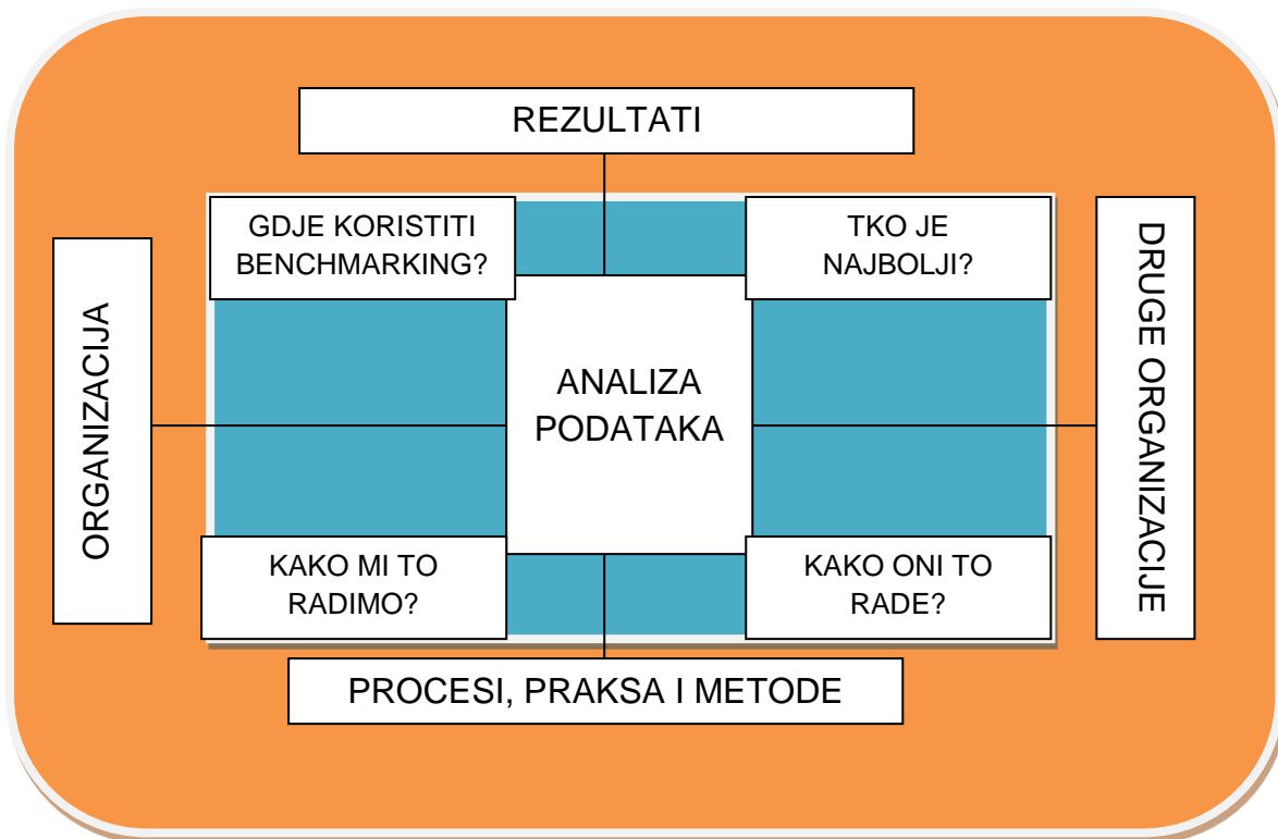
Slika 1. Koncept benchmarkinga
