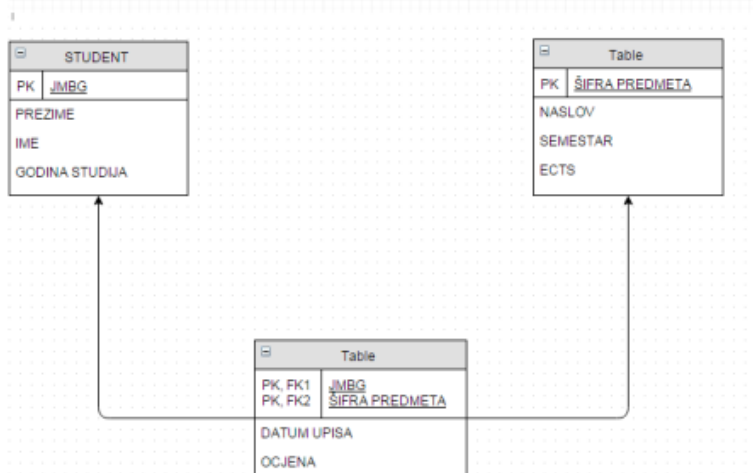
Relacijski model
