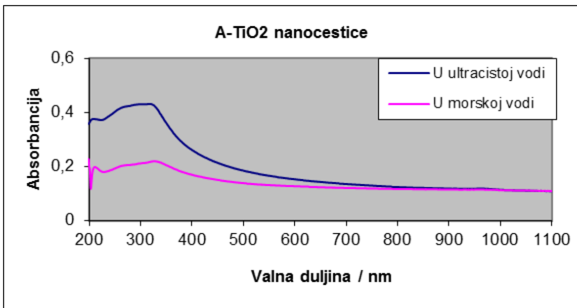
Graf 7. UV spektrofotometrijske krivulje A-TiO 2 NPs: plavom bojom prikazana je krivulja nanočestica anatsnog titanijeva(IV) oksida (100 µg/L) u ultračistoju vodi dok je ružicastom linijom prikazana krivulja istih čestica u umjetnoj morskoj vodi.
