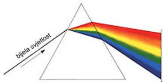
Slika 4: zraka sunčeve svjetlosti pada kroz prizmu, lomi se pod različitim kutovima, a na drugoj strani prizme stvara sunčev spektar boja ( http://www.zlatarna.com/images/slike/disperzija.jpg , 01.11.2017.)
