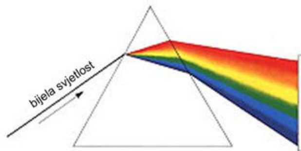
Slika 4: zraka sunčeve svjetlosti pada kroz prizmu, lomi se pod različitim kutovima, a na drugoj strani prizme stvara sunčev spektar boja
