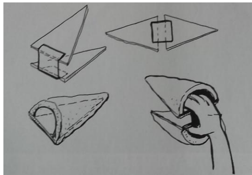
Slika 10. Izrada kljuna za životinje (Izvor: Varl, 2001:10)
