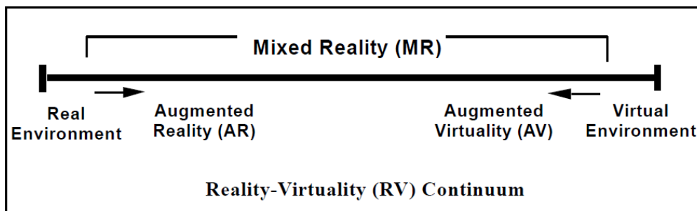
Slika 1. Virtualni kontinuum
