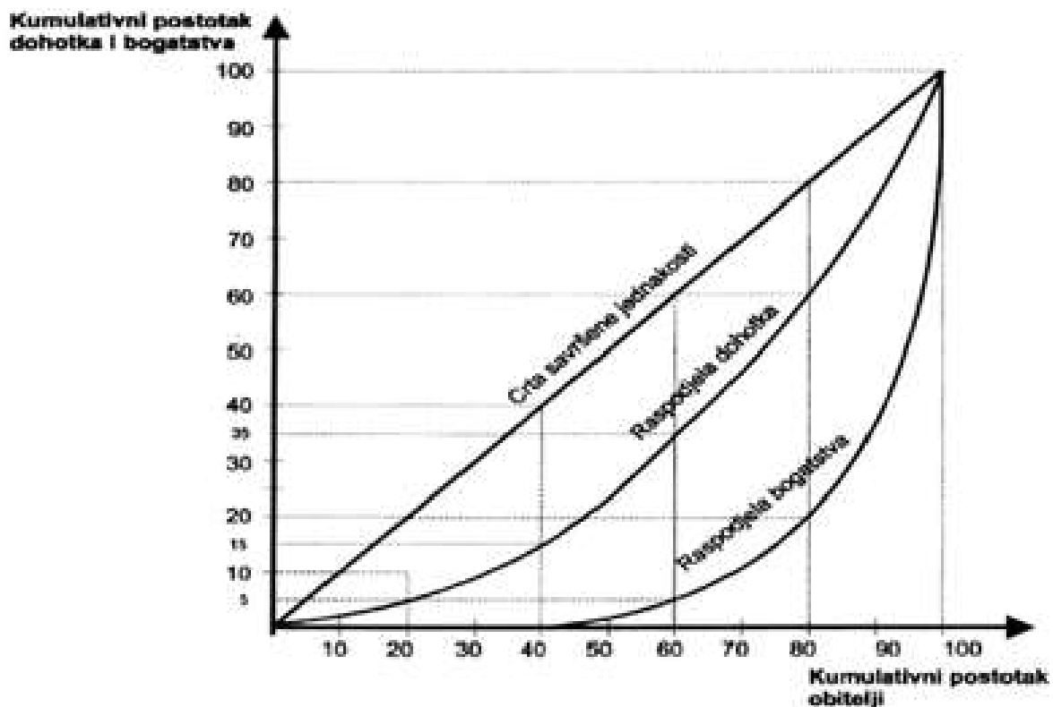
Slika 1: Lorenzova krivulja
