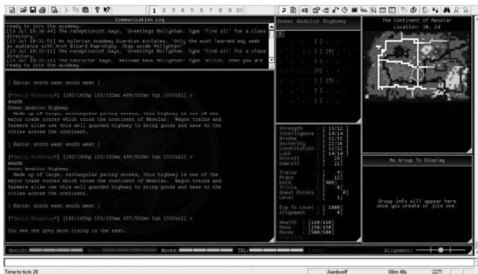
Slika 2. Aardwolf MUD [2]
