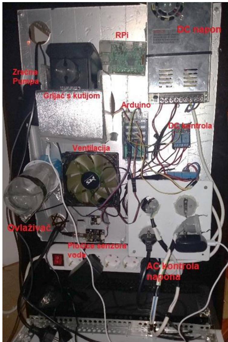
Slika 13. Vanjska strana matične ploče (Izvor: autor)
