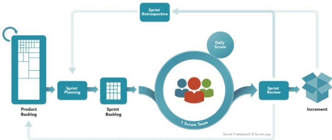
Slika 9. SCRUM
