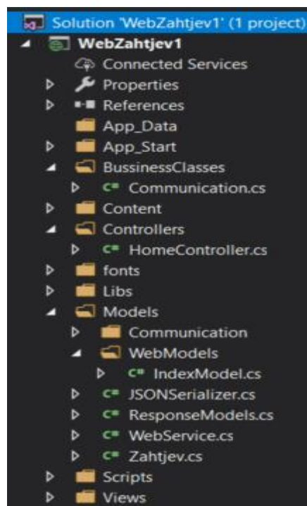
Slika 25. Komponente web aplikacije
