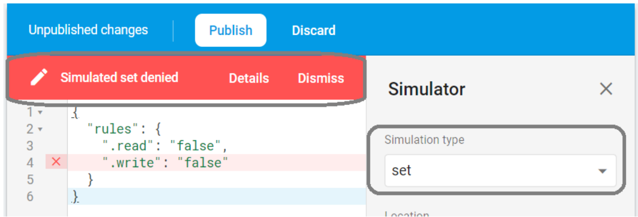
Slika 4. Prikaz rada alata za simuliranje pravila u firebase bazi podataka. Izradio: autor.
