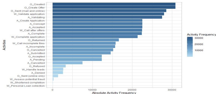
Slika 38 Histogram podataka
