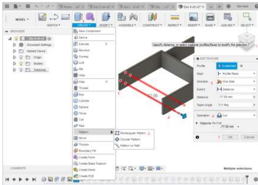
Slika 30. Kreiranje utora za pričvršćivanje dijelova robotske ruke
