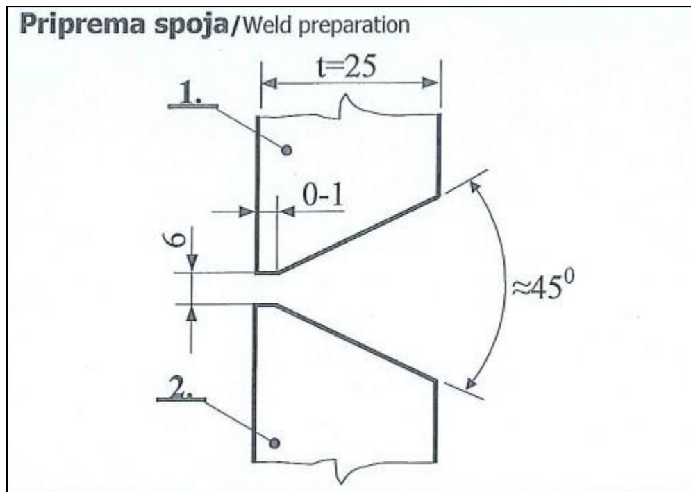
Slika 4 "V" spoj
