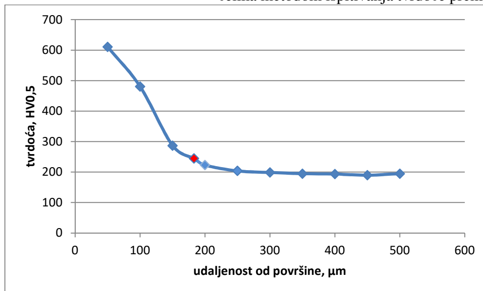
Slika 31. Ovisnost tvrdoće udaljenosti od površine za uzorak 2
