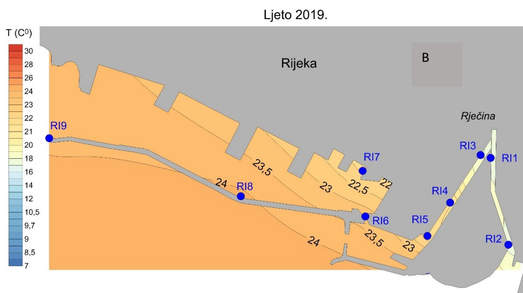
Slika 6: Raspodjela temperature mora (°C) u površinskom sloju tijekom zime 2019. (A) i ljeta 2019. (B)
