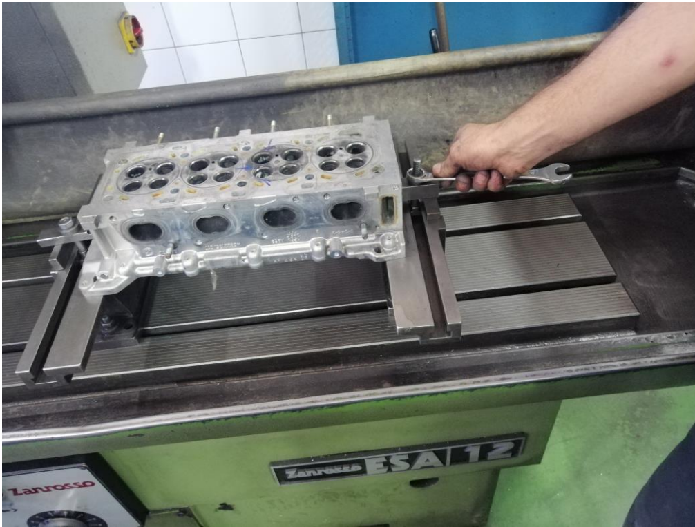
Slika 22 Pričvršćivanje držača na radni stol
