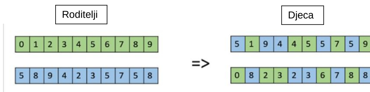
Slika 6.: Uniformno križanje
