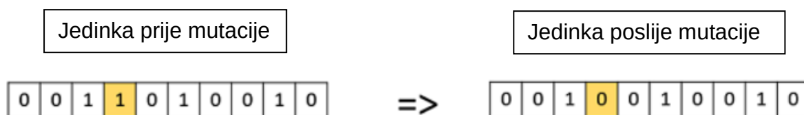
Slika 8.: Mutacija
