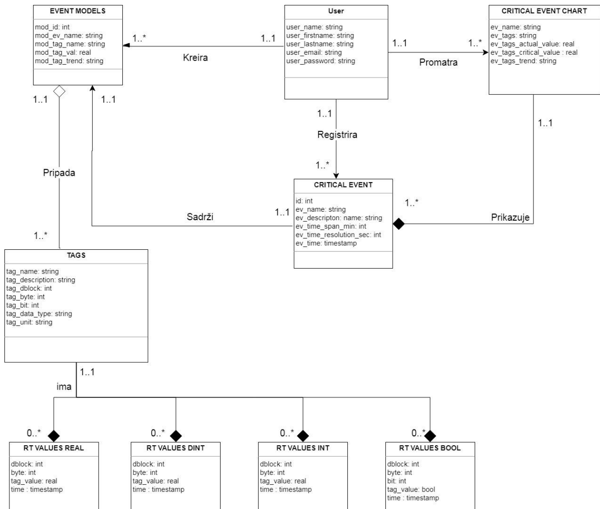
Slika 6: Klasni dijagram
