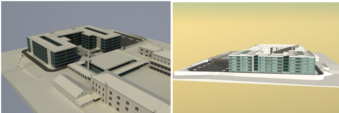
Slika 14 Simulacija adaptacije 1
