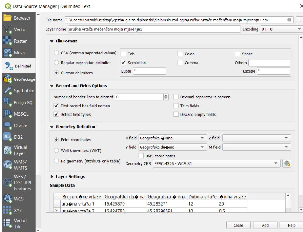
Slika 37. Delimited Text
