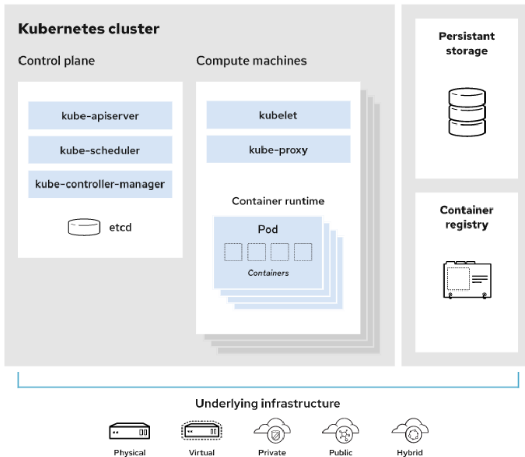
Slika 7: Kubernetes arhitektura [10]
