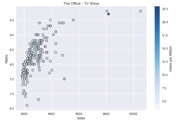
Slika 65. Dijagram raspršenja
