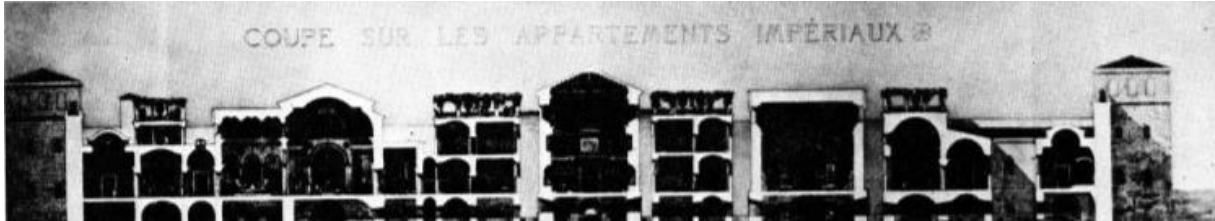
Slika 2. Presjek kroz Dioklecijanov stan
